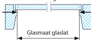
Afb. 2 – bijv. Roto-raam met schuine/rechte glaslat
