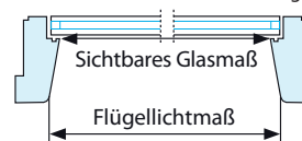
Skizze 1 – z.B. Velux-Fenster mit Schräger Glaslat
