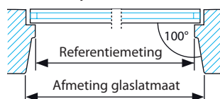
Schets 2 – bijv. Roto-raam met schuine/rechte glaslat
