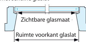
Afb. 2 – bijv. Roto-raam met schuine/rechte glaslat
