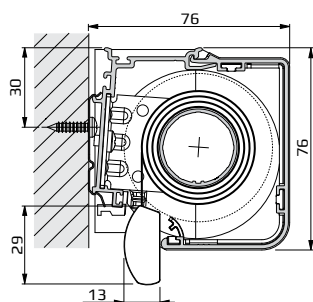
Metalen clip, gebogen, voor cassette (leveringsomvang)
