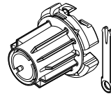
Tegenlager in hoogte verstelbaar +/- 4 mm verstelbereik, voor 38/43 mm
