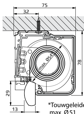
Metalen clip, gebogen, voor cassette (leveringsomvang)
