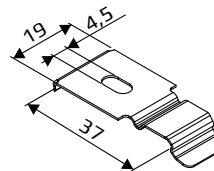
Clip voor geleideprofiel 54007 zilver (op aanvraag)
