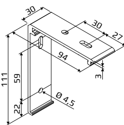
Houder voor cassette
