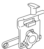
Glijder met adapter en vergrendeling voor paneeldrager B+C, kan van onderaf worden ingestoken
