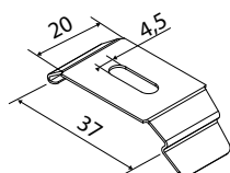
Metalen clip, gebogen, voor cassette (leveringsomvang)
